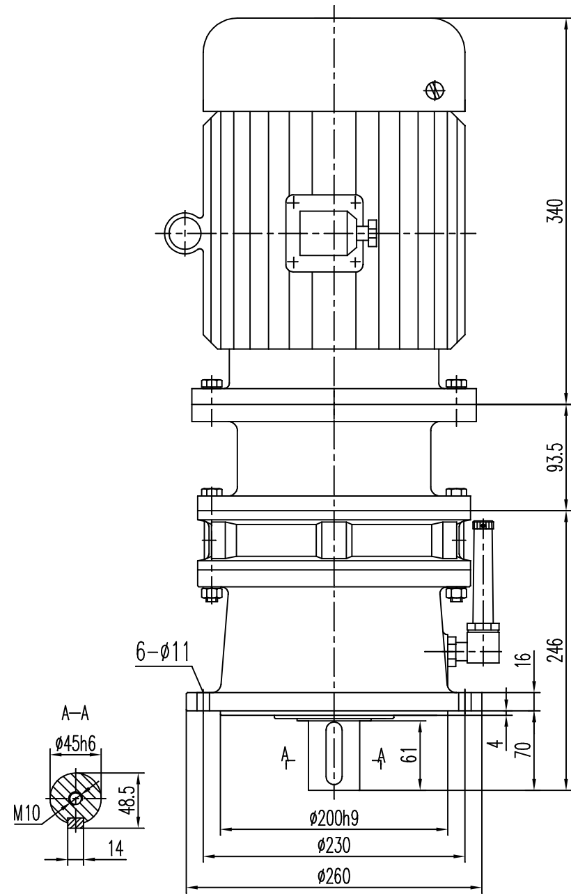
BLD2-4kw NER GROUP CO.,LIMITED 立式电机直联型摆线针轮减速机 www.sogears.com
