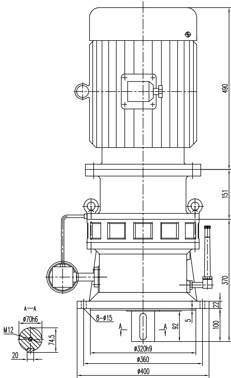
BLD4-11kw NER GROUP CO.,LIMITED 立式电机接盘型摆线针轮减速机 www.sogears.com
