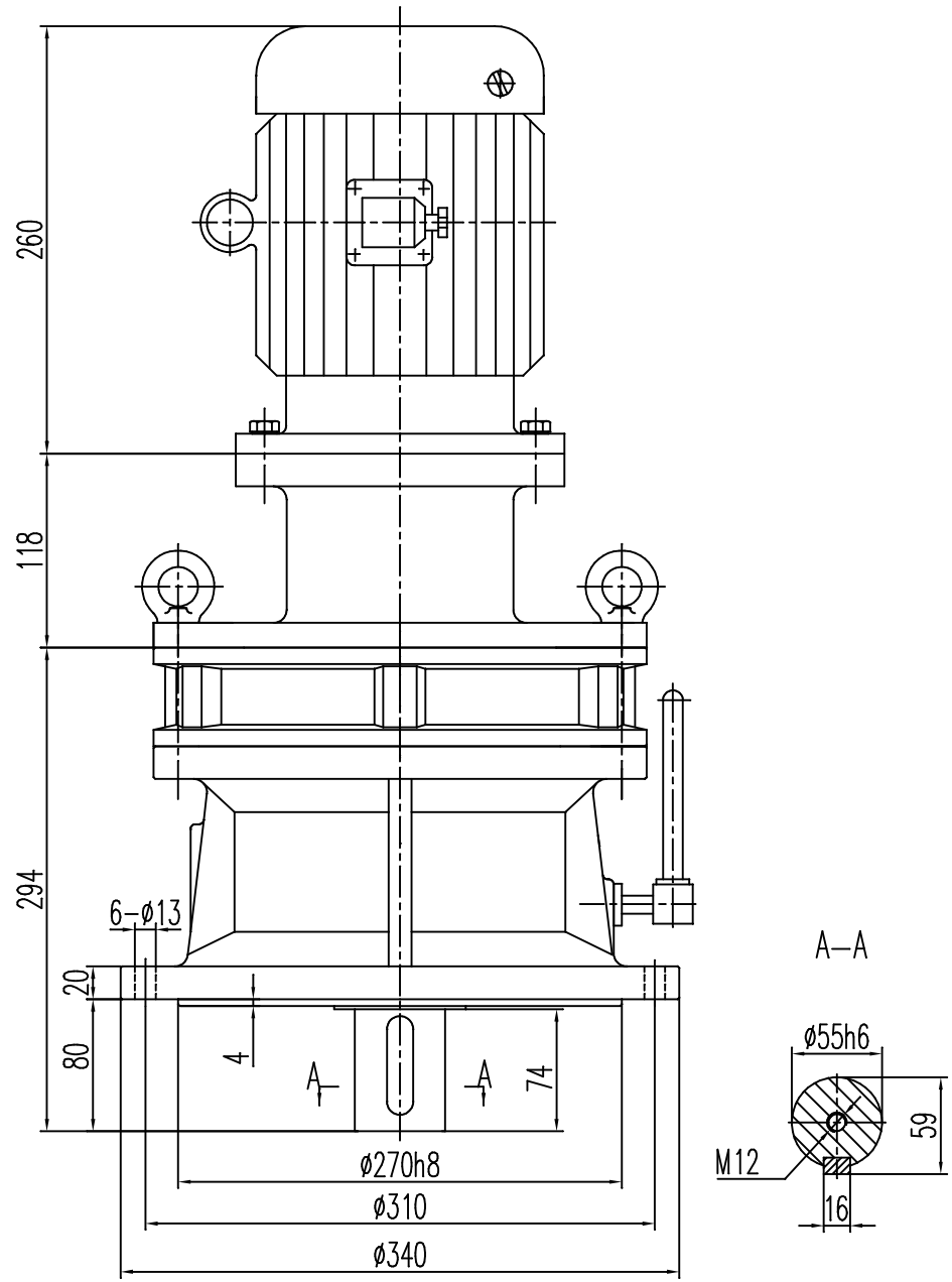
BLD3-1.1kw 立式电机接盘型摆线针轮减速机 NER GROUP CO.,LIMITED www.sogears.com
